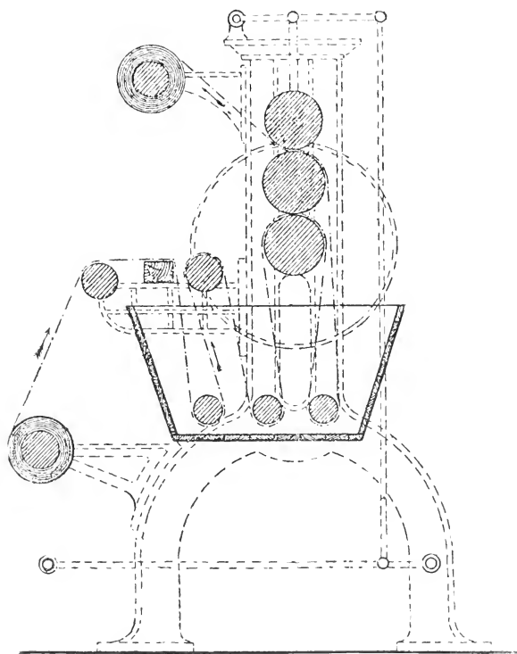
FIG. 26.—Padding Machine.
